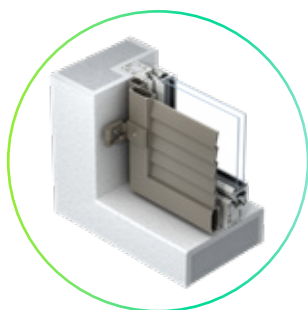
Montaggio dei cardini al telaio su serramento, non alla parete
