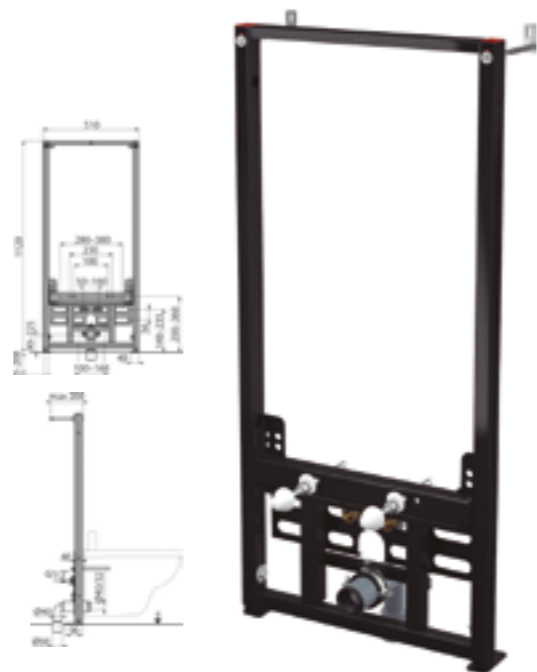
Estrutura para bidé S150/225
