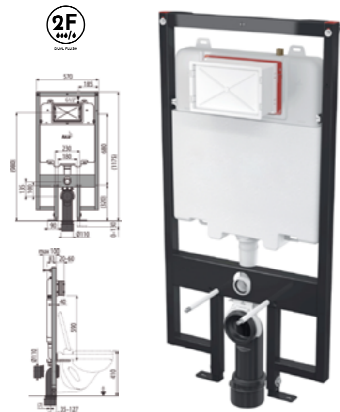
Estrutura para sanitário suspenso e ao chão S200/300 Ref.: RES110ISLM Pack: 17 kg / 0,09 m 3
