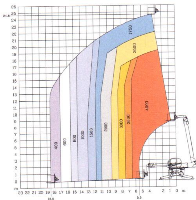
Rotation sur stabilisateurs déployés avec fourches
