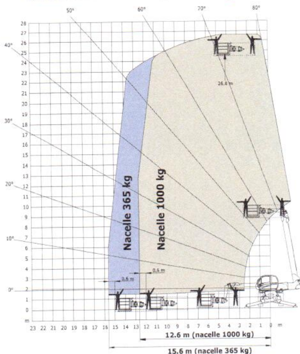
Rotation sur stabilisateurs déployés avec nacelle 365/1000 kg
