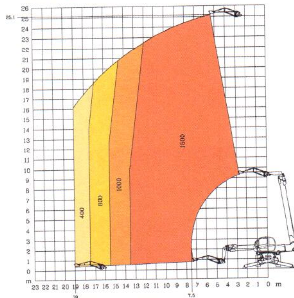
Rotation sur stabilisateurs déployés 3D positif / négatif
