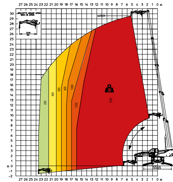
JW 1500 potence avec treuil 1.500
