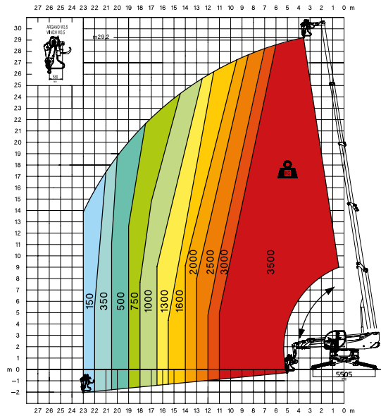
W 3,5 crochet 3,5 tonnes
