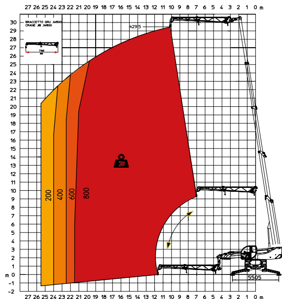
JW 800 potence avec treuil 800
