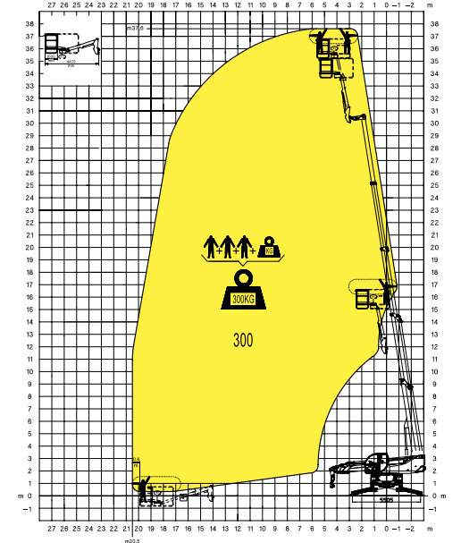
TP O-U nacelle télescopique pivotante positif-négatif avec rotation 340°
