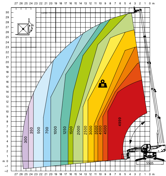
Abaque de charge sur stabilisateurs déployés en rotation avec fourches
