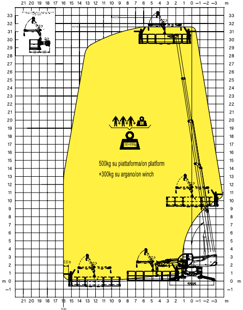
TP O-U nacelle télescopique pivotante positif-négatif avec rotation 340°
