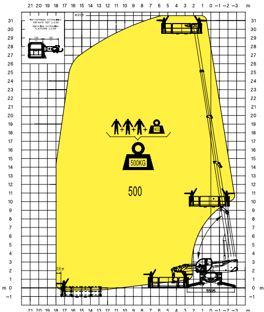
TP Plateforme télescopique TP
