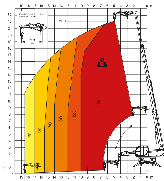
JW 2000 potence avec treuil 2.000
