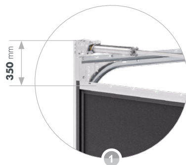
Linéau min. 350 mm
