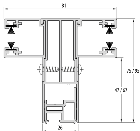
• Rail de division RGT 75/95 • Roka top 2 RG / RG EX
