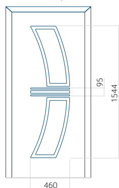
Dessin technique
