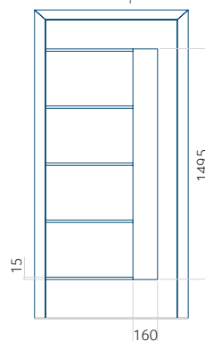
Dessin technique
