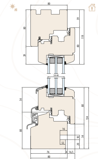
SYSTÈME NATURO 80 découpe pour l'appui de fenêtre intérieur
