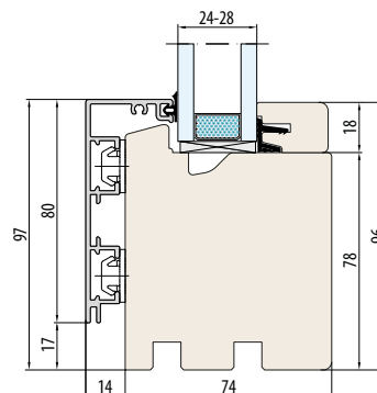
SYSTÈME ESPERIA LIFE 74 ALU-Fix
