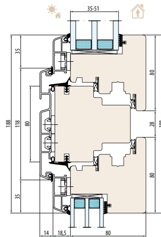
SYSTÈME NATURO 80 GEMINI CLASSIC traverse 80 mm
