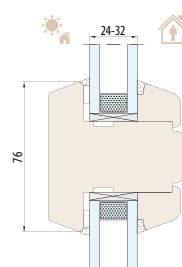
SYSTÈME NATURO 68 meneau structurel 76 mm
