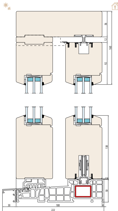
SYSTÈME NATURO 80 HST (dimensions générales) - seuil 50 mm - schéma "C"
