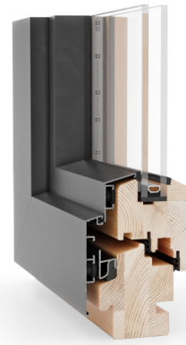
Profil Reno Line (à rainure)
