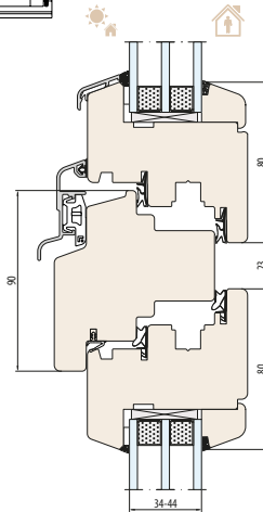
SYSTÈME NATURO 80 traverse 90 mm
