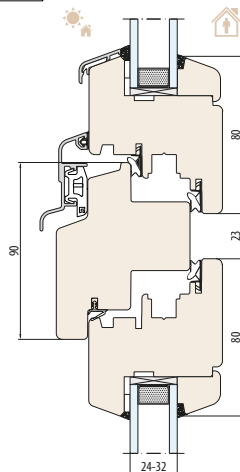
SYSTÈME NATURO 68 traverse 90 mm
