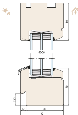
SYSTÈME NATURO 92-Fix découpe pour l'appui de fenêtre extérieure
