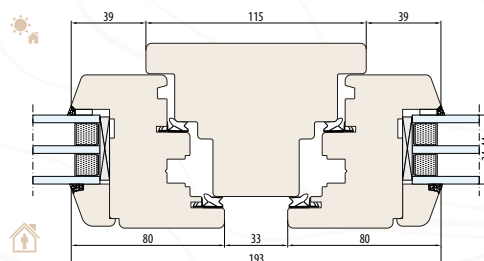
SYSTÈME NATURO 80 meneau fixe 115 mm (section horizontale)
