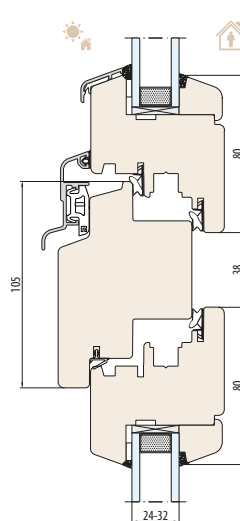
SYSTÈME NATURO 68 traverse 105 mm
