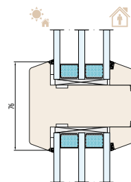
SYSTÈME NATURO 92 meneau structurel 76 mm
