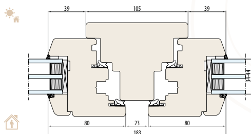
SYSTÈME NATURO 80 meneau fixe 105 mm (section horizontale)
