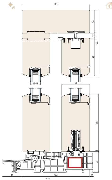
SYSTÈME NATURO 68 HST (dimensions générales) - seuil 50 mm - schéma "C"
