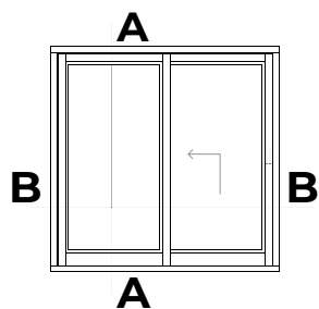
SYSTÈME NATURO 68 HST (dimensions générales) - seuil 22 mm - schéma "A"
