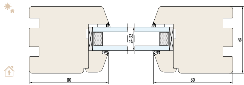
SYSTÈME NATURO 68-Fix SECTION HORIZONTALE B-B
