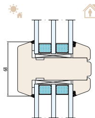
SYSTÈME NATURO 92 meneau structurel 68 mm
