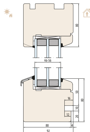
SYSTÈME NATURO 92-Fix découpe pour l'appui de fenêtre intérieur
