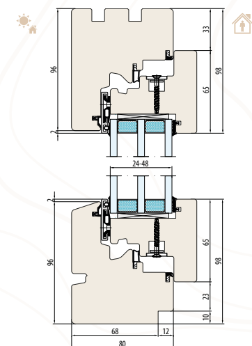
SYSTÈME ESPERIA LIFE 80 découpe pour l'appui de fenêtre intérieur
