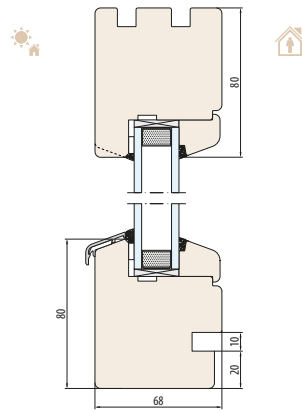
SYSTÈME NATURO 68-Fix découpe pour l'appui de fenêtre intérieur
