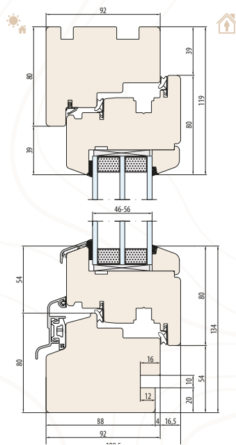
SYSTÈME NATURO 92 découpe pour l'appui de fenêtre intérieur
