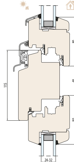
SYSTÈME NATURO 68 traverse 115 mm
