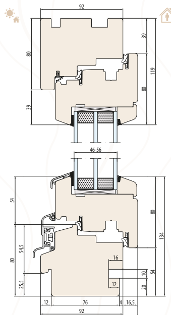
SYSTÈME NATURO 92 découpe pour l'appui de fenêtre intérieur et extérieur
