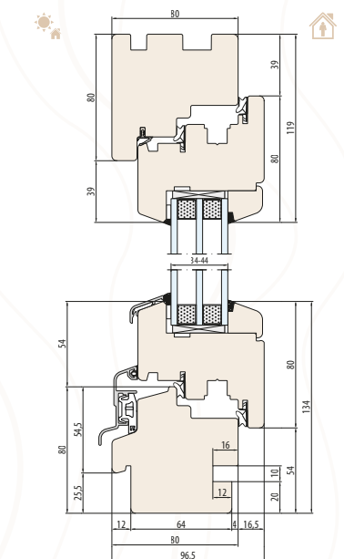
SYSTÈME NATURO 80 découpe pour l'appui de fenêtre intérieur et extérieur
