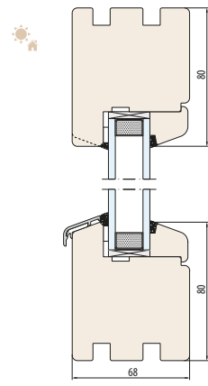
SYSTÈME NATURO 68-Fix sans découpe pour l'appui de fenêtre
