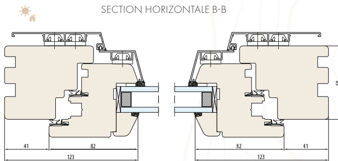
SYSTÈME NATURO 68 ALU RENO LINE
