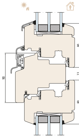
SYSTÈME NATURO 92 traverse 90 mm
