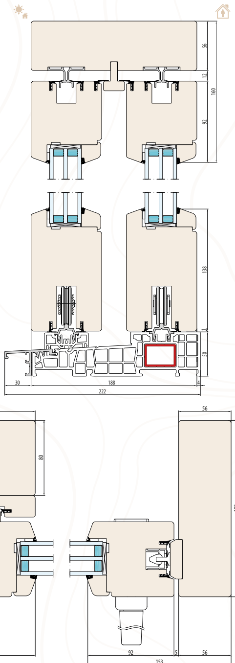
SYSTÈME NATURO 80 HST (dimensions générales) - seuil 50 mm - schéma "D"
