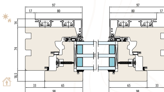
SYSTÈME ESPERIA LIFE 74 ALU SECTION HORIZONTALE B-B
