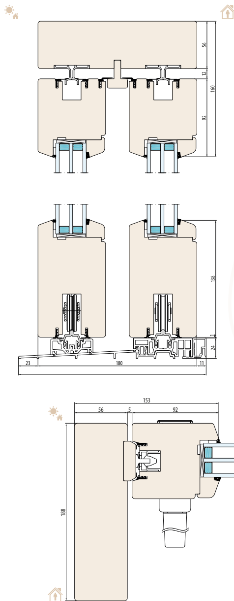
SYSTÈME NATURO 80 HST (dimensions générales) - seuil 24 mm - schéma "D"
