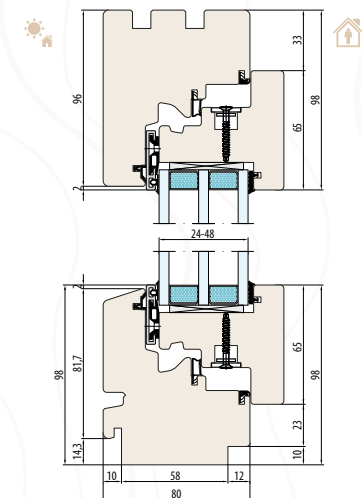
SYSTÈME ESPERIA LIFE 80 découpe pour l'appui de fenêtre intérieur et extérieur
