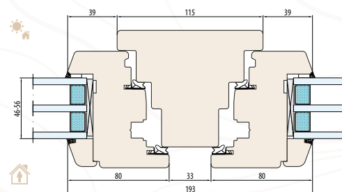
SYSTÈME NATURO 92 meneau fixe 115 mm (section horizontale)
