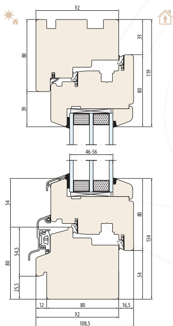
SYSTÈME NATURO 92 découpe pour l'appui de fenêtre extérieur
