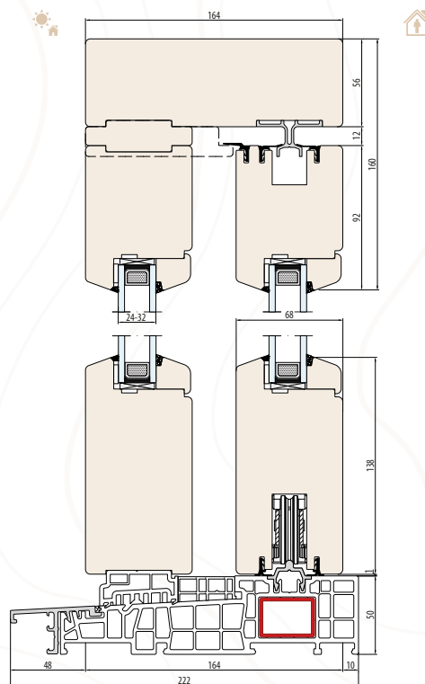
SYSTÈME NATURO 68 HST (dimensions générales) - seuil 50 mm - schéma "A"
