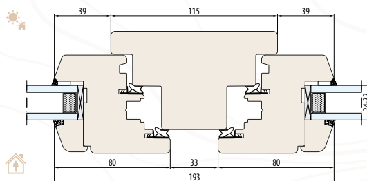
SYSTÈME NATURO 68 meneau fixe 115 mm (section horizontale)
