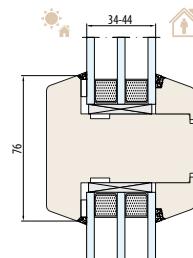
SYSTÈME NATURO 80 meneau structurel 76 mm
