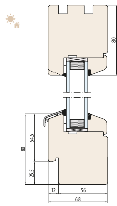
SYSTÈME NATURO 68-Fix découpe pour l'appui de fenêtre extérieur
