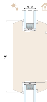
SYSTÈME NATURO 68 meneau structurel 140 mm
