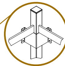
Detalle de columna en esquina. Details of the corner column. Détail colonne sur coin.
