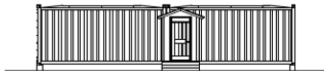
JULKISIVU ITÄÄN, RAK.A
