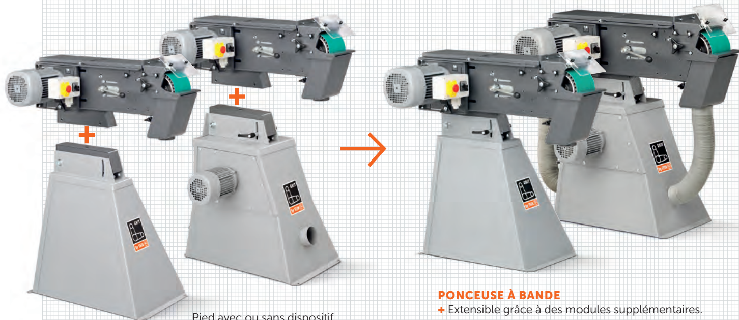
Pied avec ou sans dispositif d'aspiration pour les poussières de ponçage GIB / GIBE
