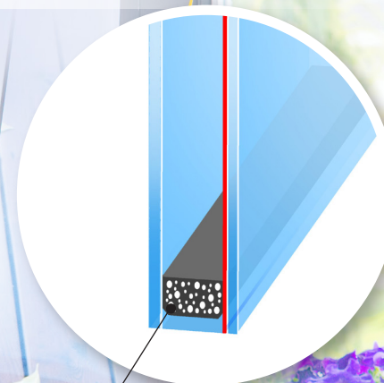
Intercalaire classique ou Warm edge
