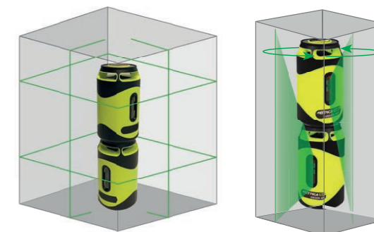
BEISPIELE FÜR 2 GESTAPELTE FLASH 360°, 2 VERTIKALE BELIEBIG EINSTELLBARE LASER
