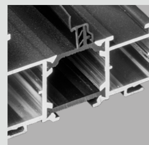
Bouclier thermique sur le dormant (en option Premio et Equilibre)
