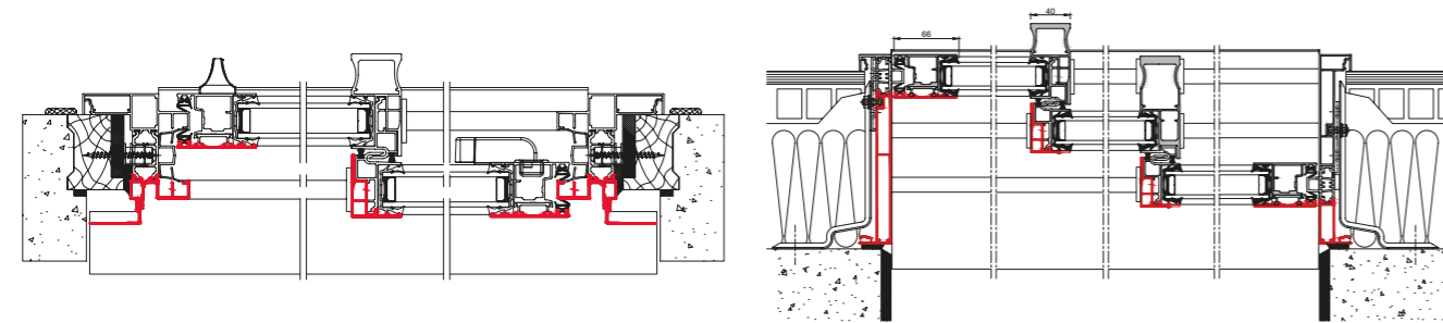
Baie coulissante 2 rails 2 vantaux (réno)
