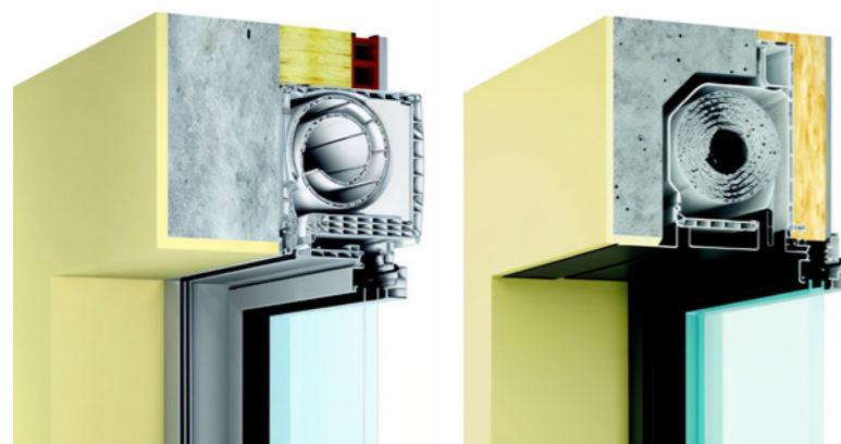
Volet roulant visible par l'intérieur
