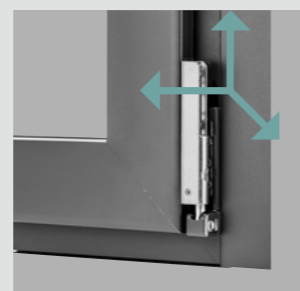
Réglage tri-dimensionnel du palier d'angle : réglage latéral, en hauteur et en compression
