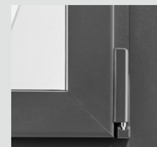
Couvre-joint intérieur aligné avec le dormant
