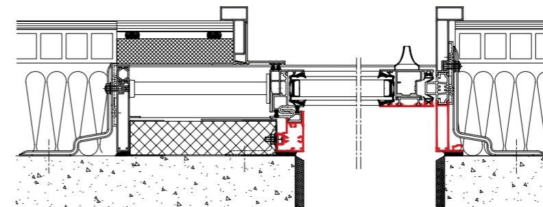
Baie à galandage 1 rail 1 vantail
