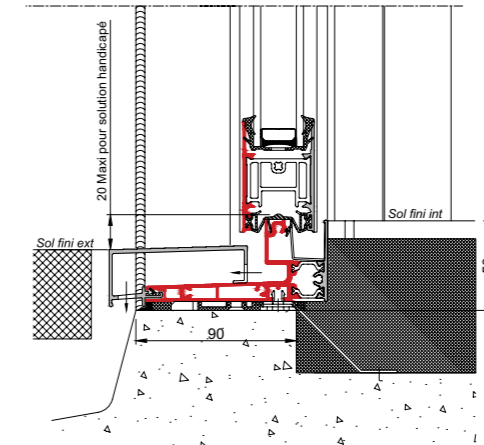
Profil d'Aménagement Extérieur (option)
