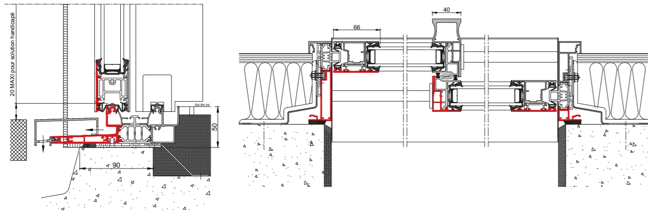
Seuil PMR (seuil encastré) et option Profil d'Aménagement Extérieur (PAE)
