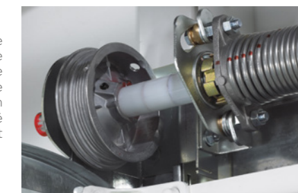
Ressort de torsion haute résistance sur axe de 25,4 mm avec sécurité ressort
