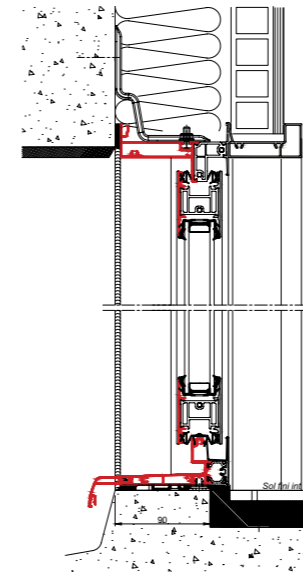
Baie à galandage 1 rail
