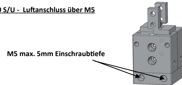
08.04.01 S/U - Über Bodenplatte anschliessbar, parallel aufgebohrt
