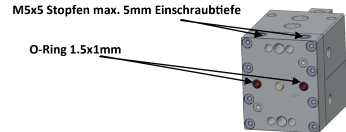
08.04.01 S/U - Über Bodenplatte anschliessbar, diagonal aufgebohrt
