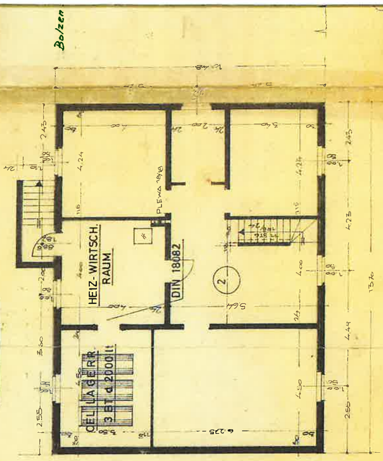
KELLERGECHOSS
