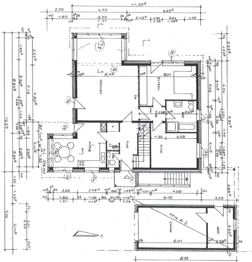
ERDGESCHOSS
