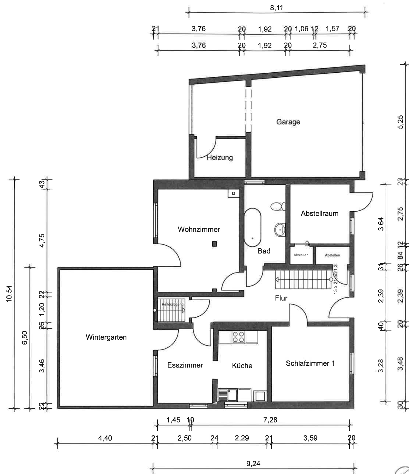
Erdgeschoss
