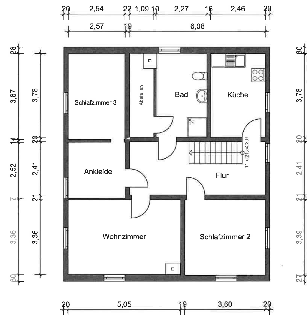
Obergeschoss
