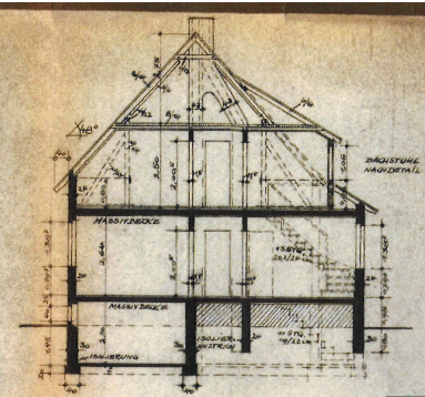
SCHNITT.
