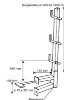
VESIKATTOKAITEET, KIINTEÄT
