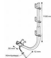
HARJAKATTOKAITEET
