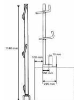
PINTA-ASENNUSKAITEET
