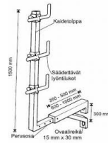
VESIKATTOKAITEET, SÄÄDETTÄVÄT
