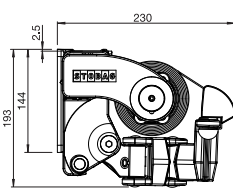
Wandmontage ohne Schutzdach Montage en façade sans auvent
