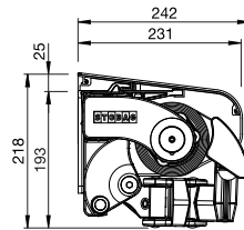
Wandmontage mit Schutzdach Montage en façade avec auvent
