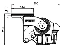
Deckenmontage ohne Schutzdach Montage sous dalle sans auvent
