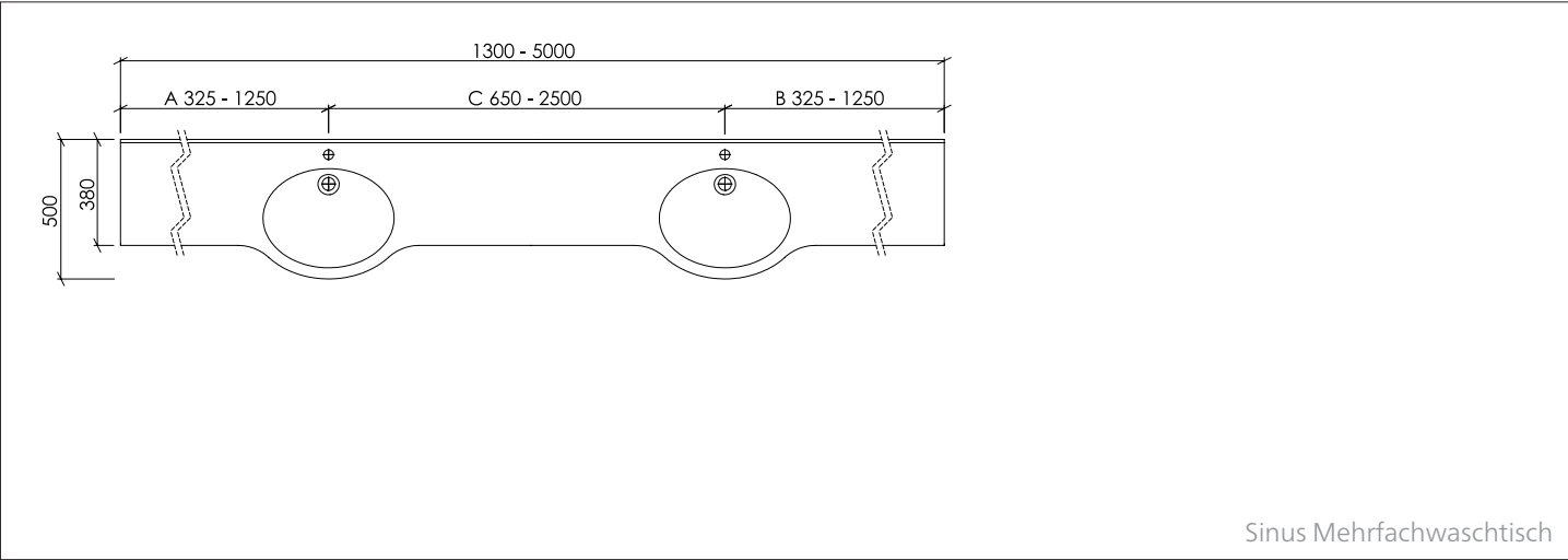
Sinus Einzelwaschtisch
